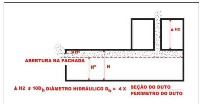
Figura 16: Diâmetro hidráulico
