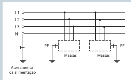
Eletrodos distintos
