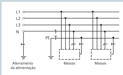
Eletrodo comum
